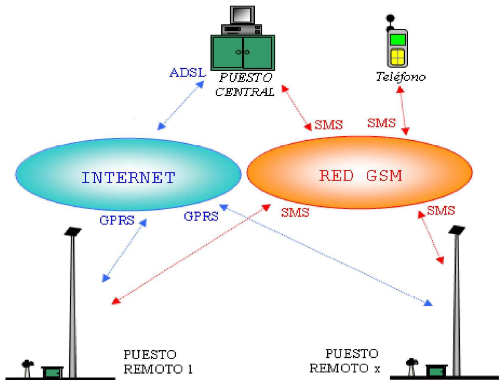
Figura 1. Filosofía de telecomunicación GSM/GPRS de Riegosalz
